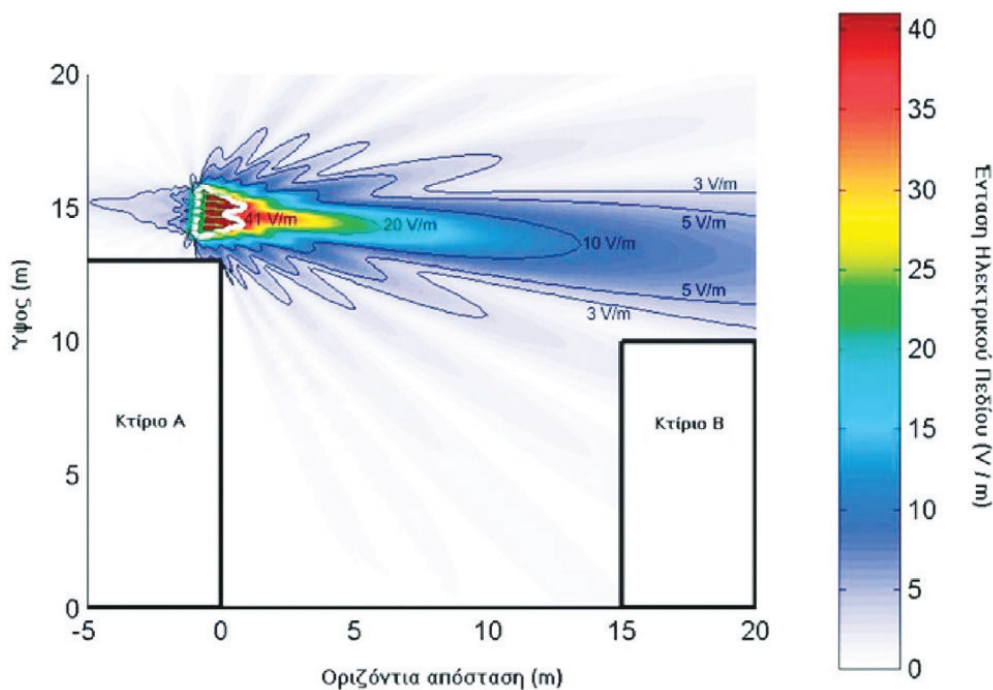
σχ.2 Διάχυση ακτινοβολίας από κεραίες.
