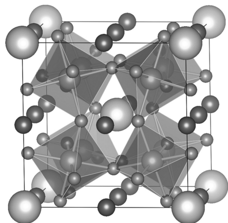
Κρυσταλλική δομή ενός περοβσκίτη, κατάλληλου για επίστρωση φωτοβολταϊκών πάνελ
